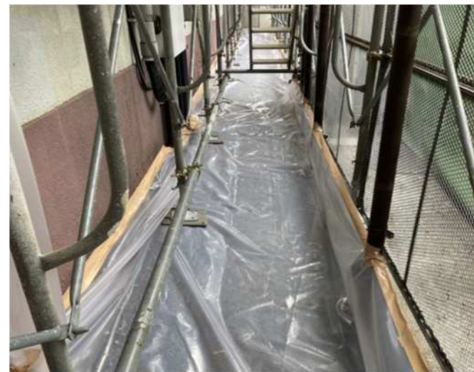
③ 飛散防止養生 (外部)
