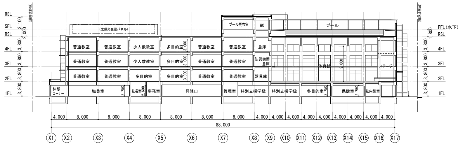
A 断面図
