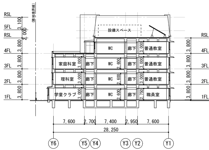
B 断面図
