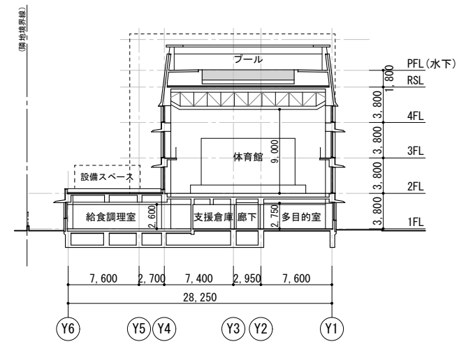
D 断面図
