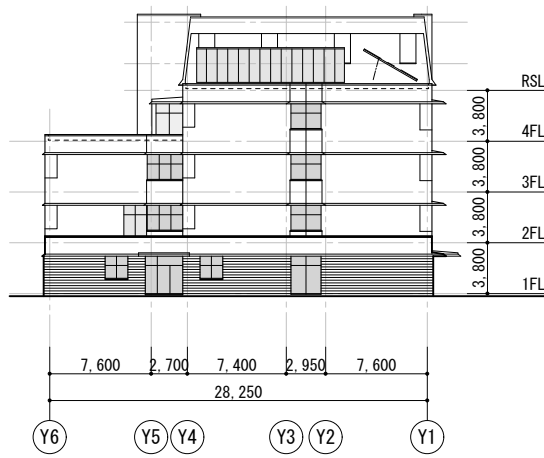
西側立面图
