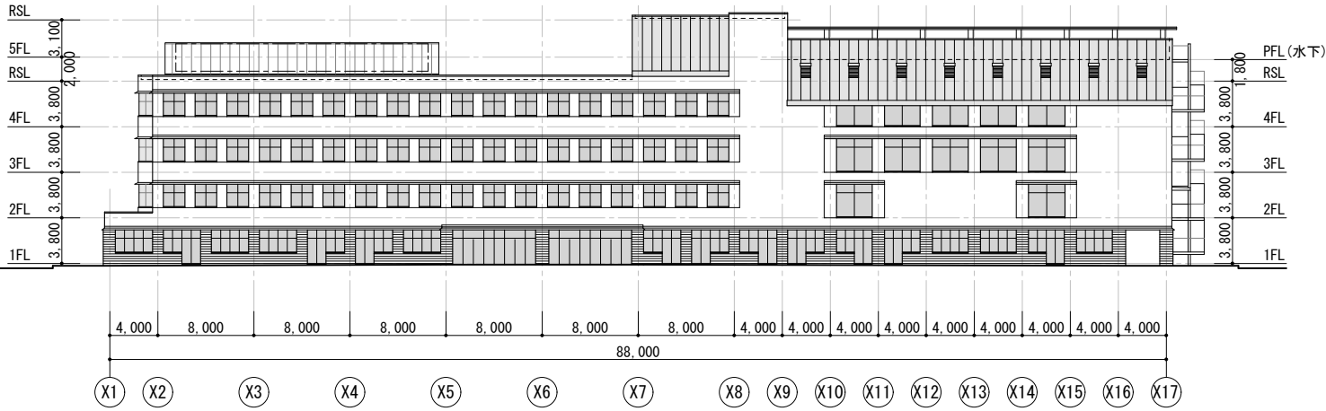
南側立面图
