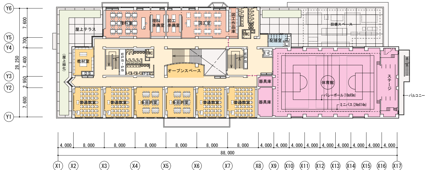
2階平面図
