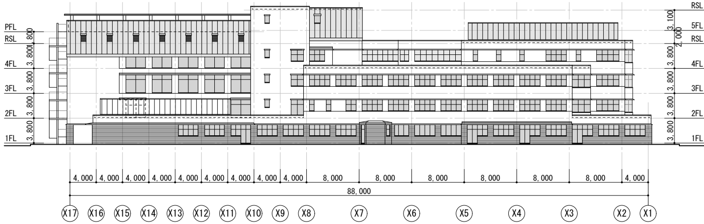
北側立面图
