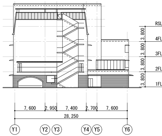
東側立面图
