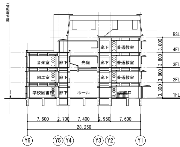
C 断面図
