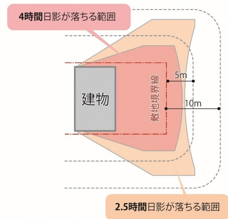
等時間日影のイメージ（平面図）
