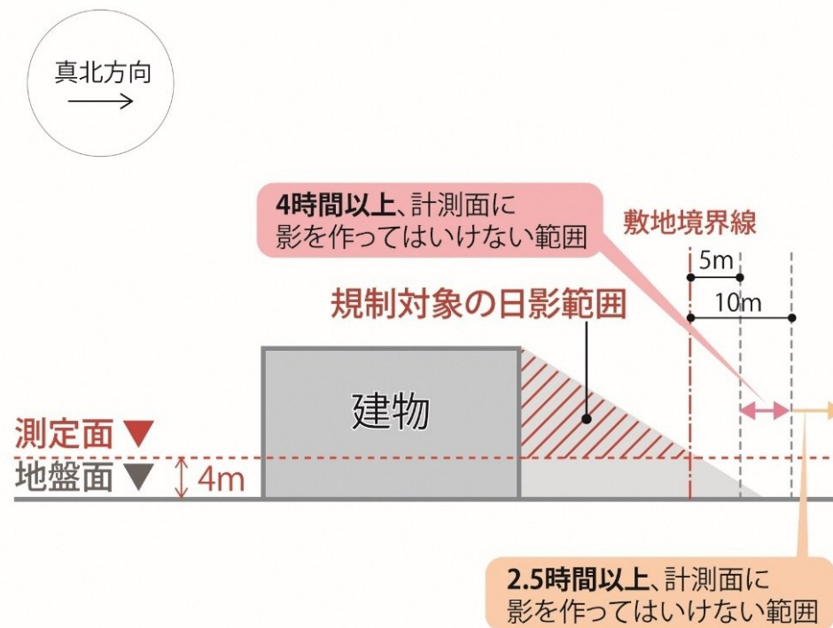
日影規制の考え方（立面図）
