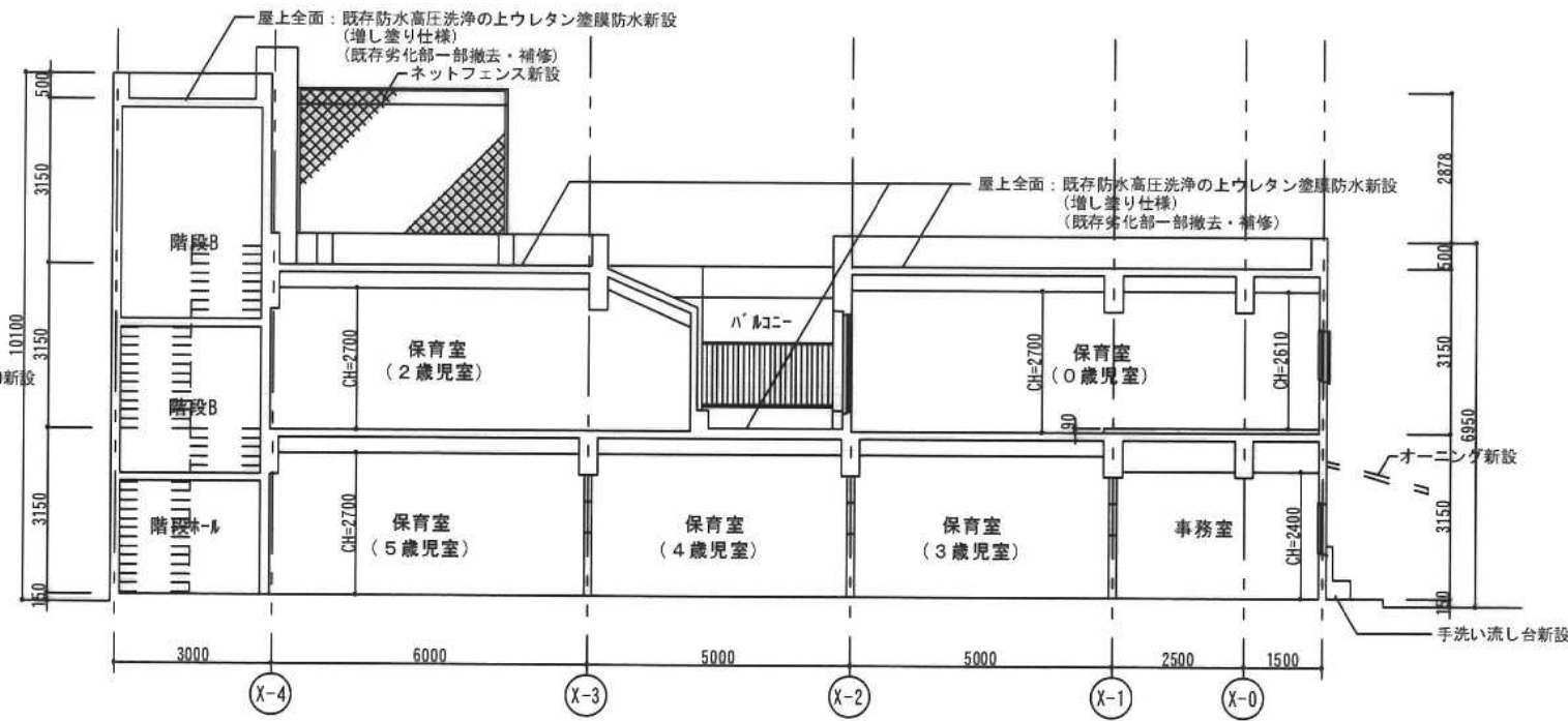
断面図 4
