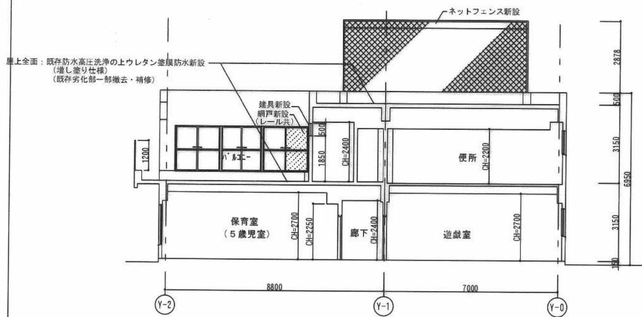
断面図 1
