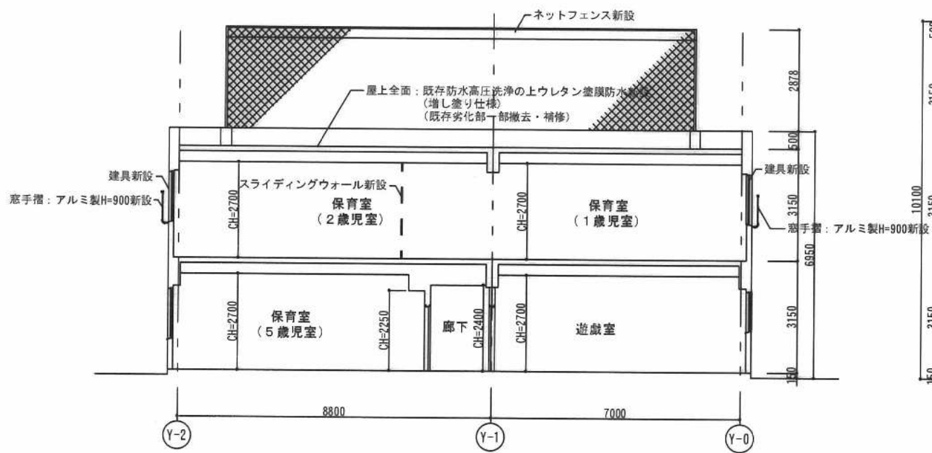
断面図 3
