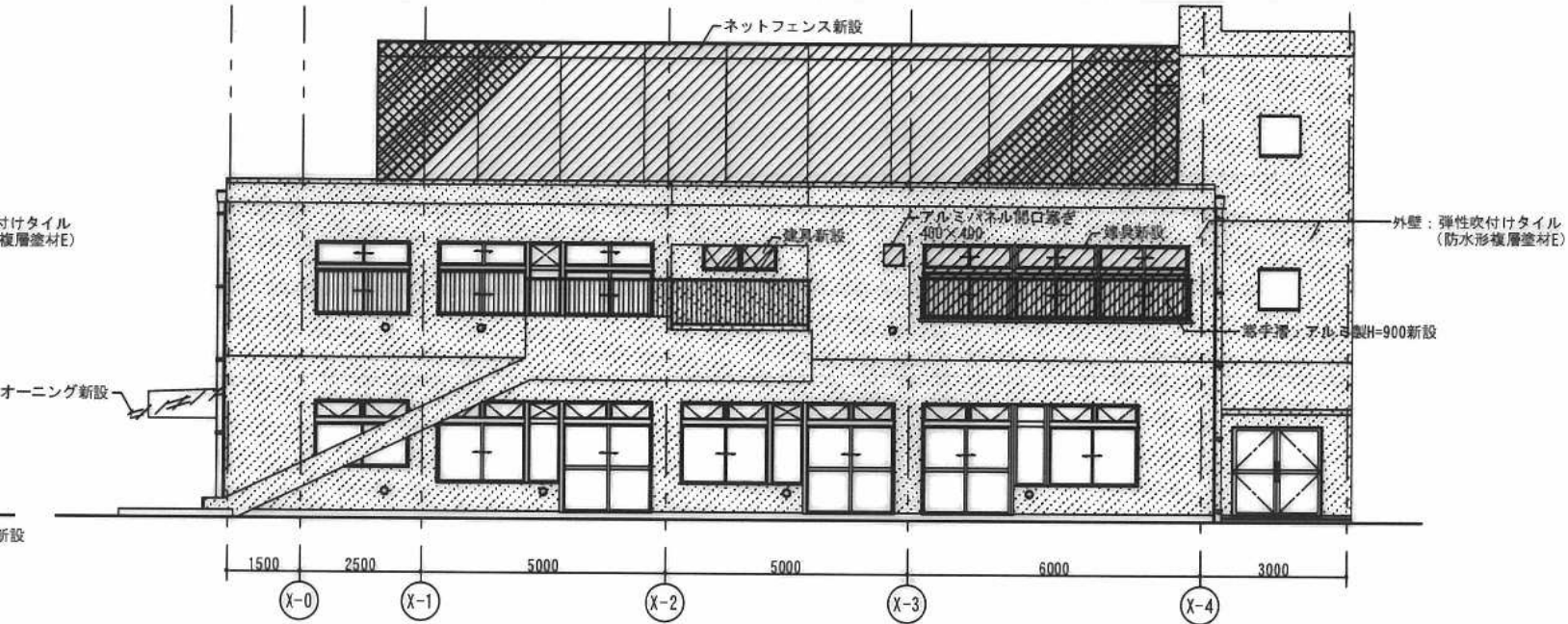
西南側立面図
