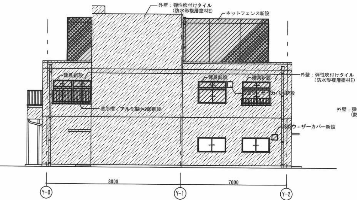
東南側立面図
