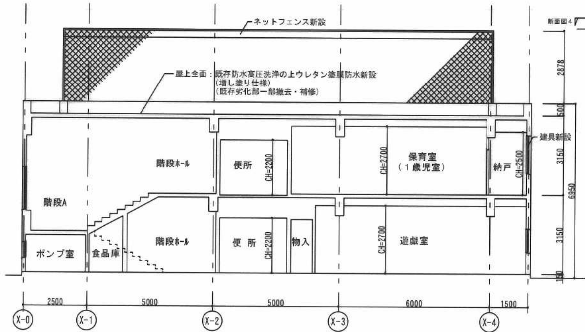
断面図 2
