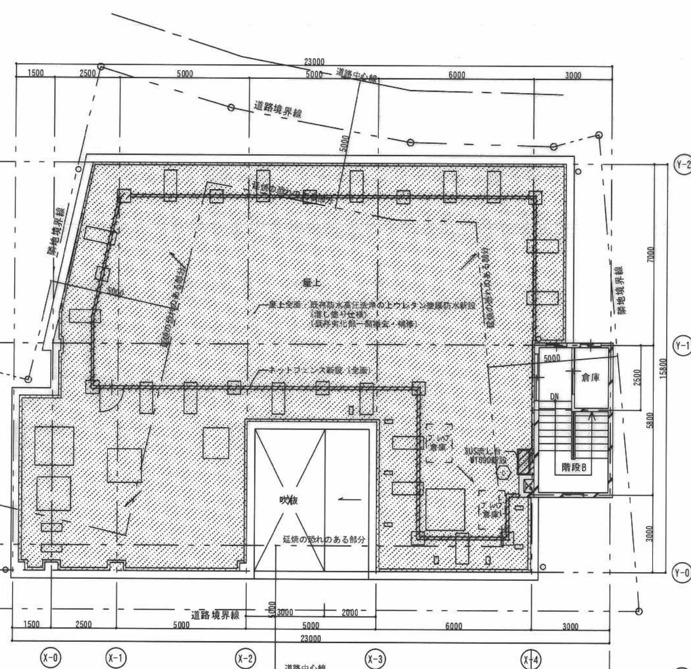
屋上階平面図
