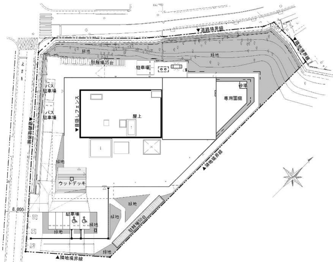
配置図 S≒1/800
