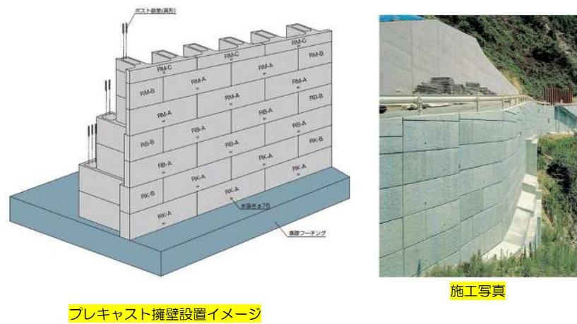
プレキャスト擁壁設置イメージ
