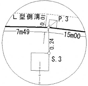
P.3、S.3 詳細図
